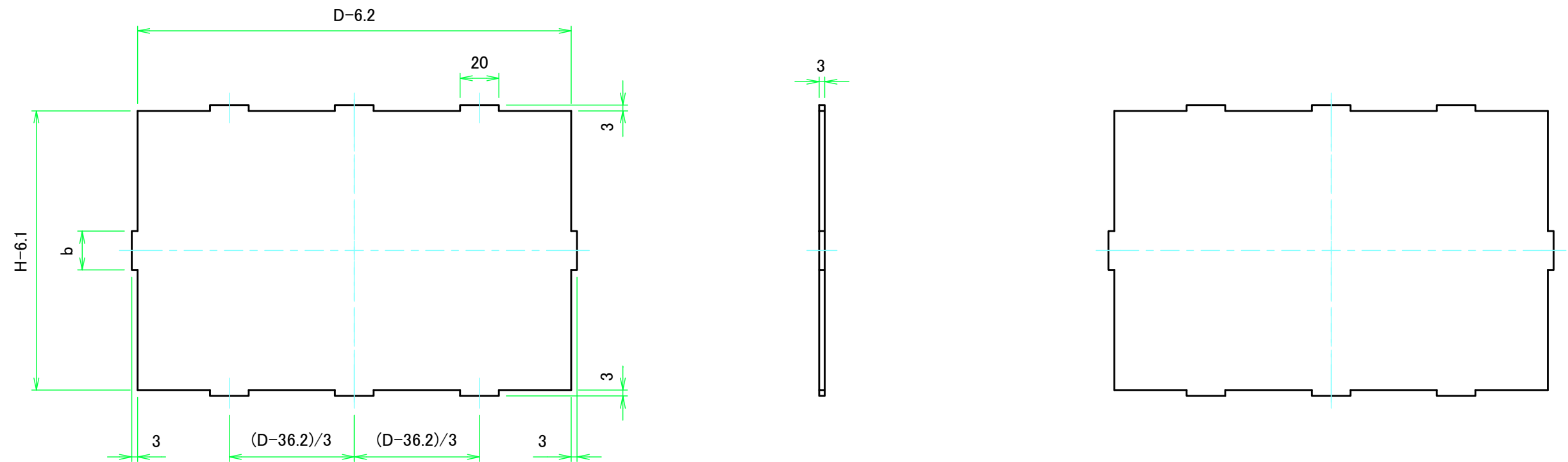
Dパネル1表面 / D panel 1 Frontside
