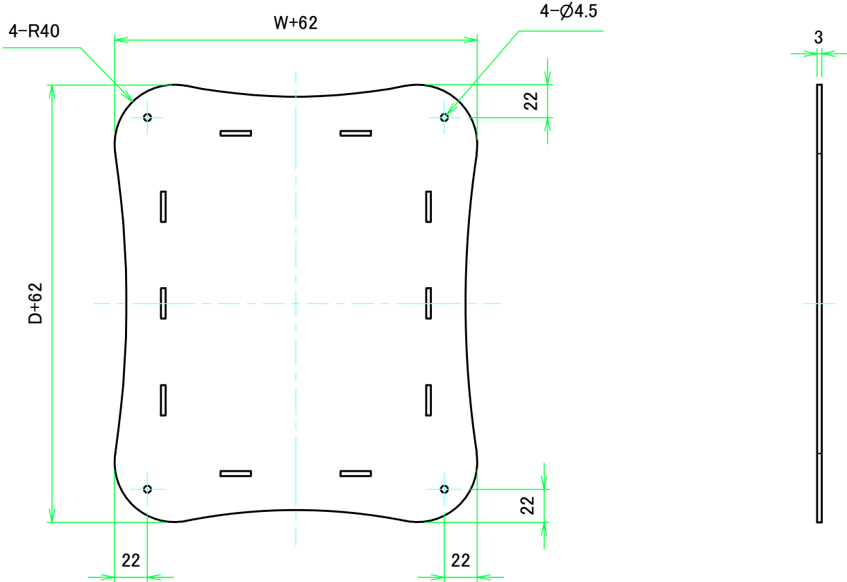
上カバー表面 / Top cover Frontside
